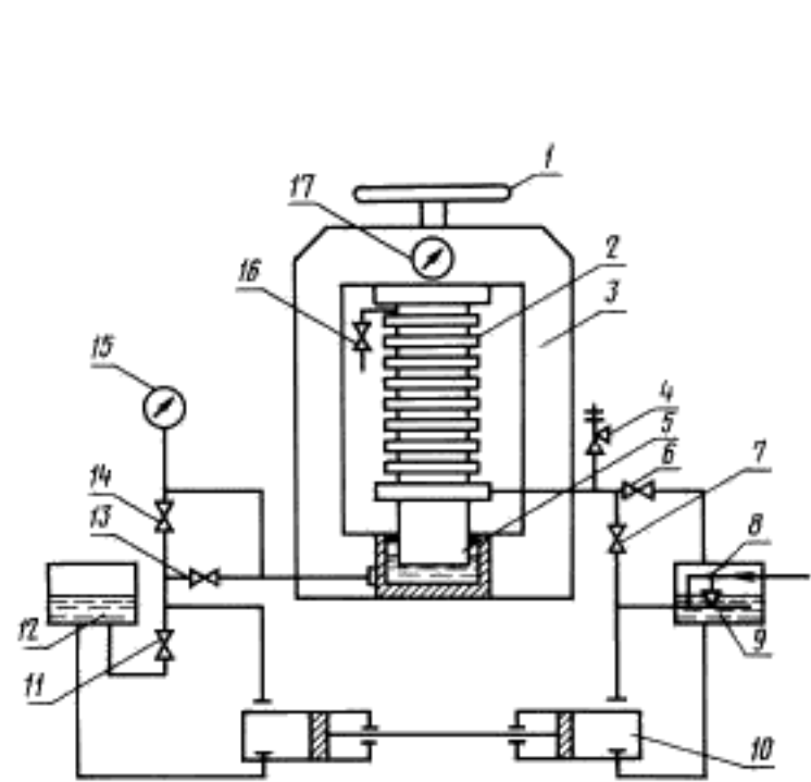
Схема автоклава АП-2
