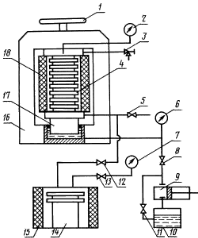
Схема автоклава типа АП-1
